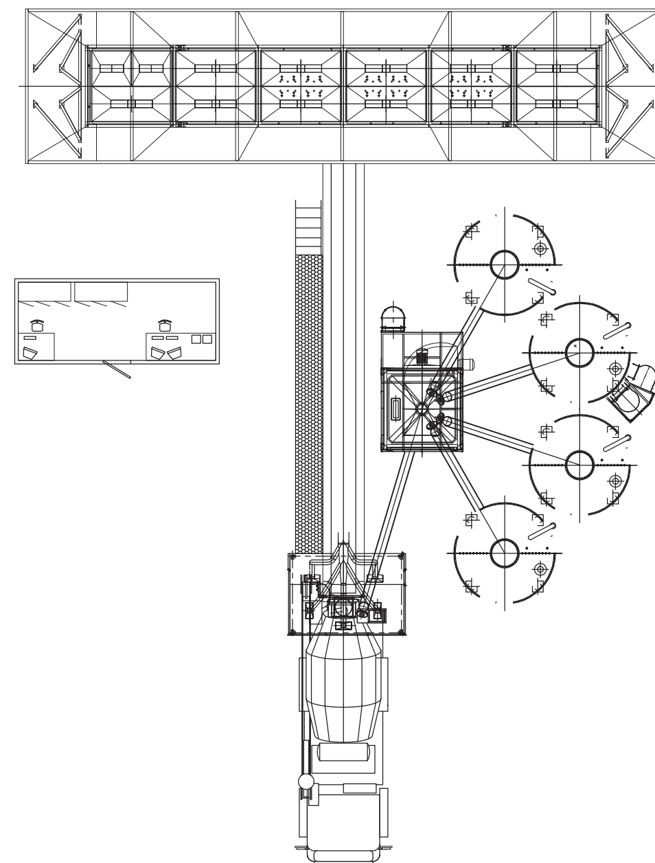
SOLUZIONE CON SCARICO CENTRALE SOLUTION WITH CENTRAL OUTPUT
