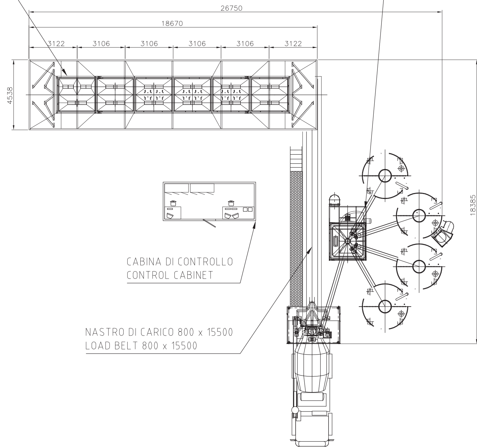
SOLUZIONE CON SCARICO LATERALE SOLUTION WITH LATERAL OUTPUT
