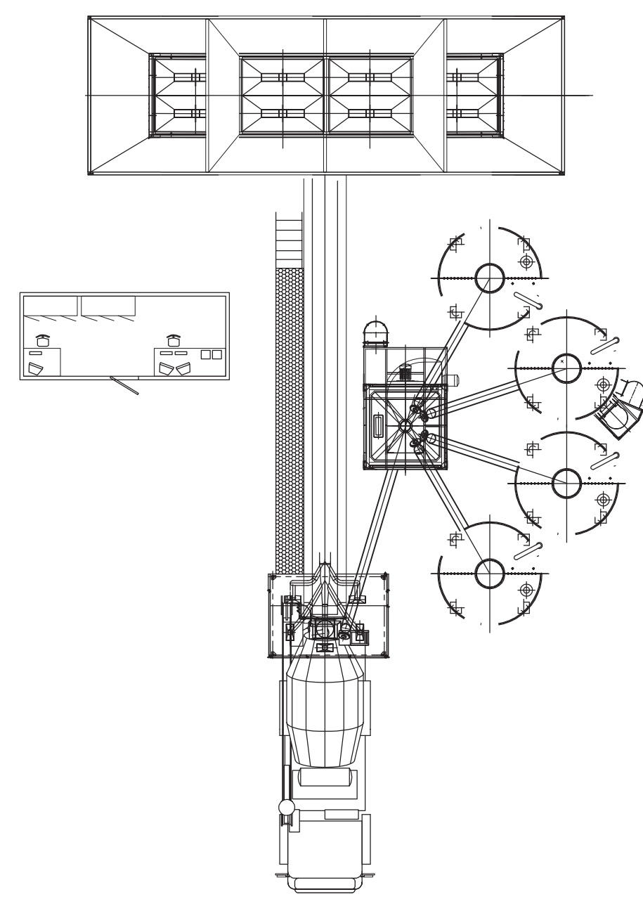
SOLUZIONE CON SCARICO CENTRALE SOLUTION WITH CENTRAL OUTPUT
