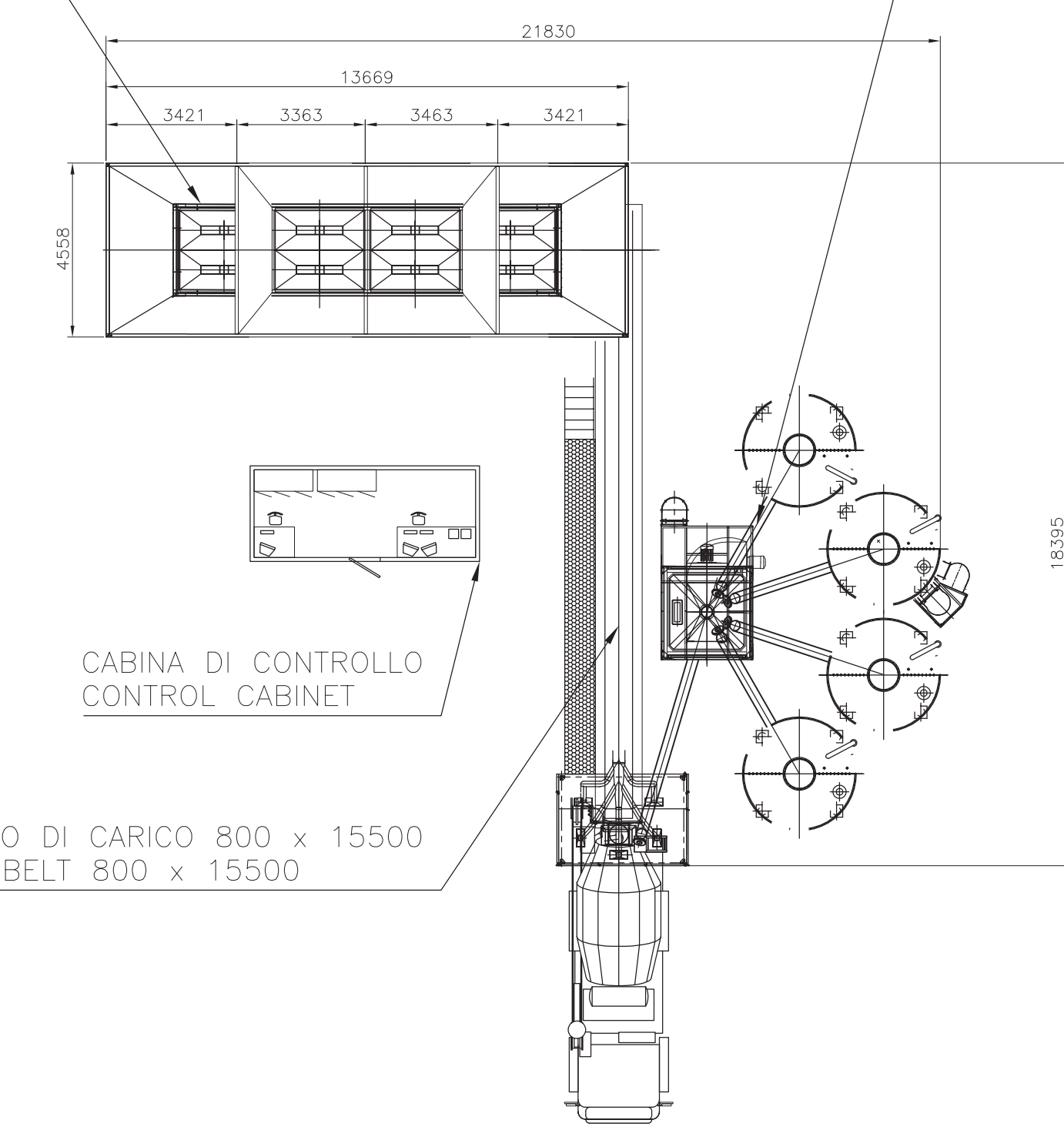
SOLUZIONE CON SCARICO LATERALE SOLUTION WITH LATERAL OUTPUT
