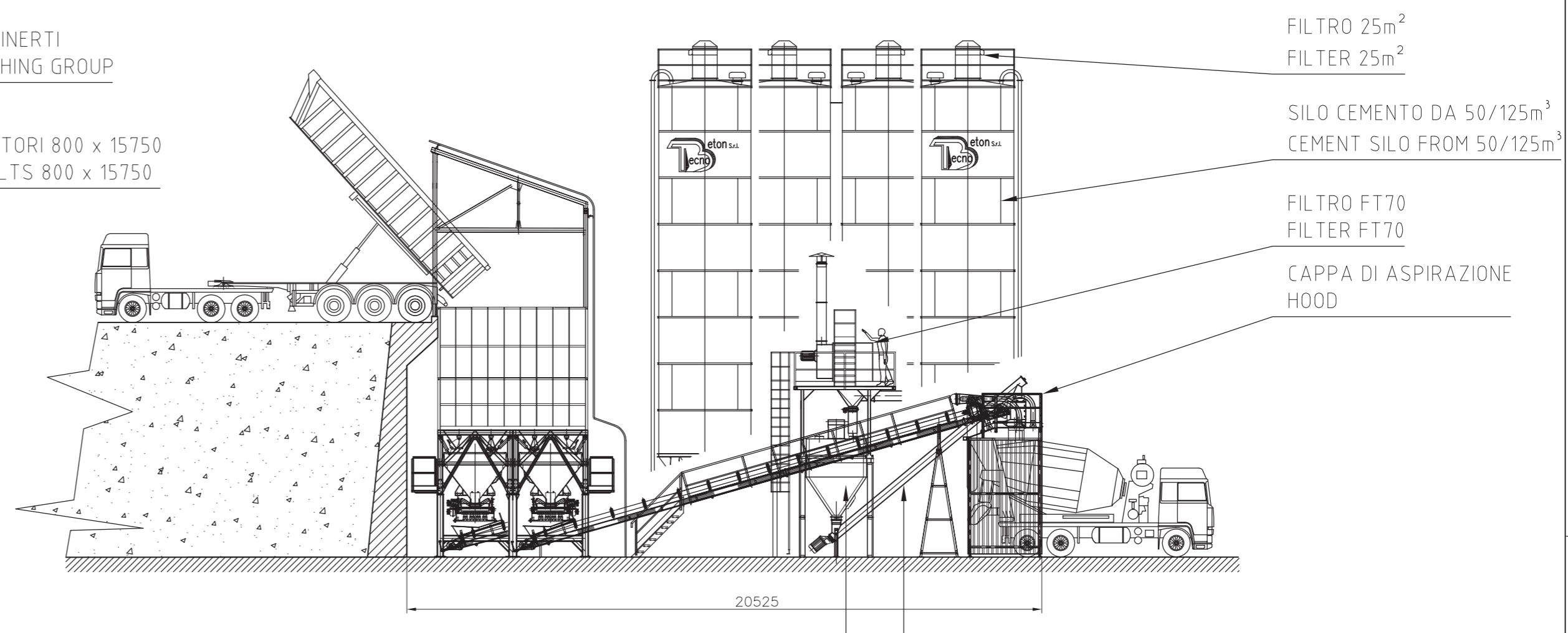
COCLEA DOSAGGIO Ø273 x 5300 SCREW CONVEYOR Ø273 x 5300
