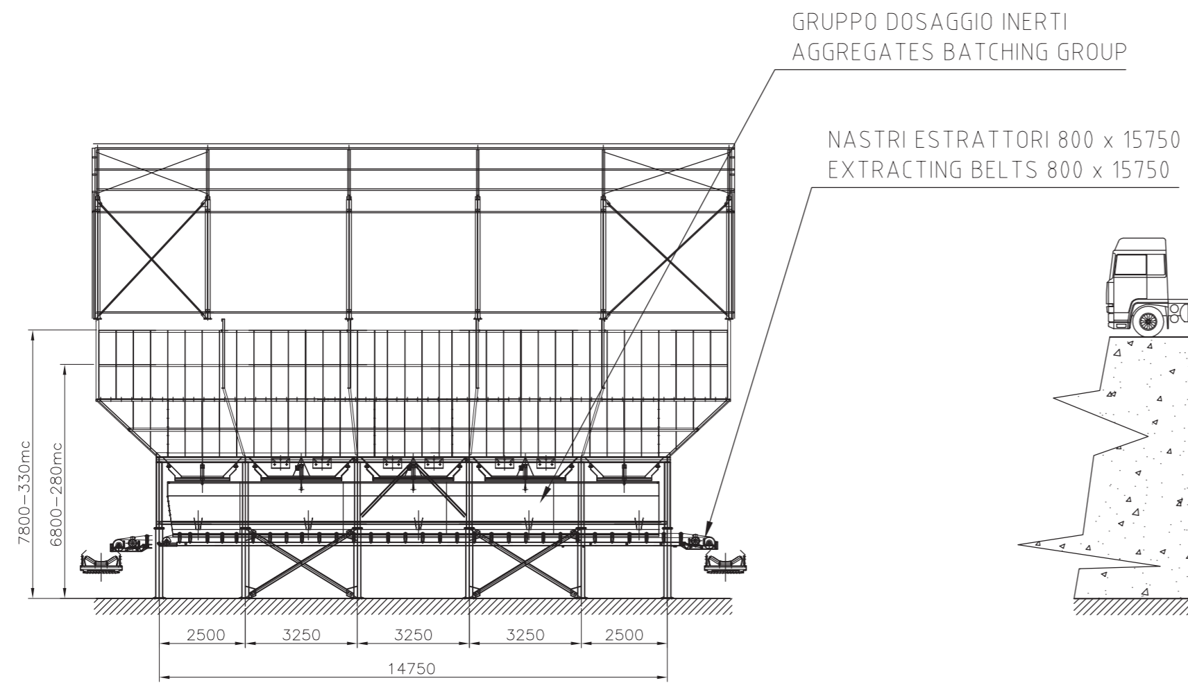
GRUPPO STOCCAGGIO INERTI DA 280/330m 3 AGGREGATES STORAGE GROUP FROM 280/330m 3
