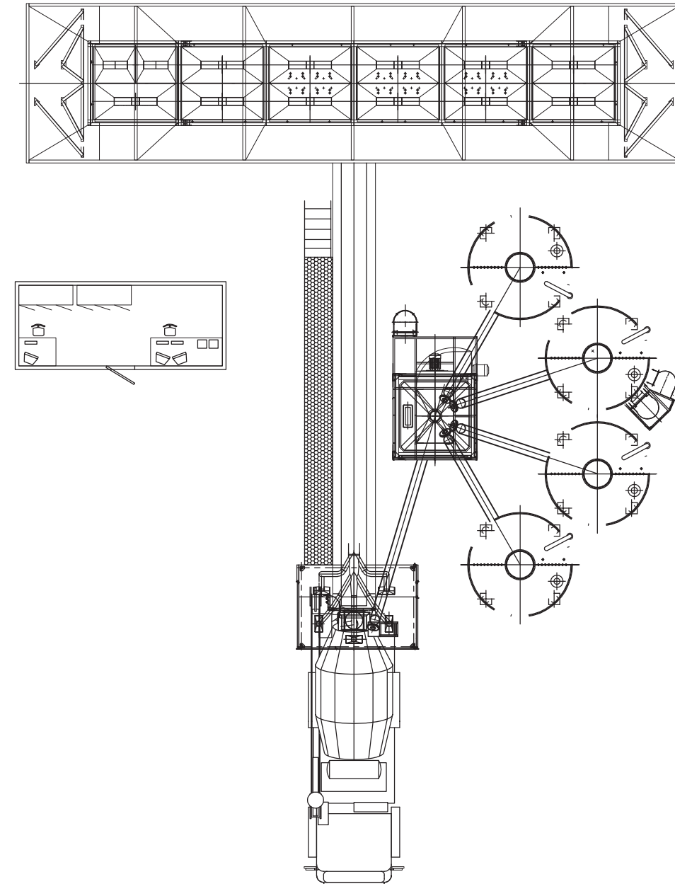
SOLUZIONE CON SCARICO CENTRALE SOLUTION WITH CENTRAL OUTPUT
