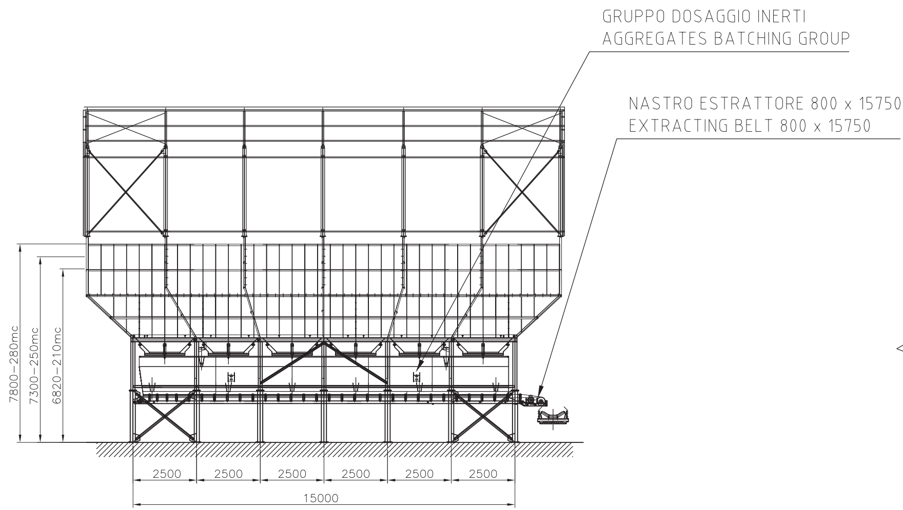
GRUPPO STOCCAGGIO INERTI DA 210/250/280m 3 AGGREGATES STORAGE GROUP FROM 210/250/280m 3
